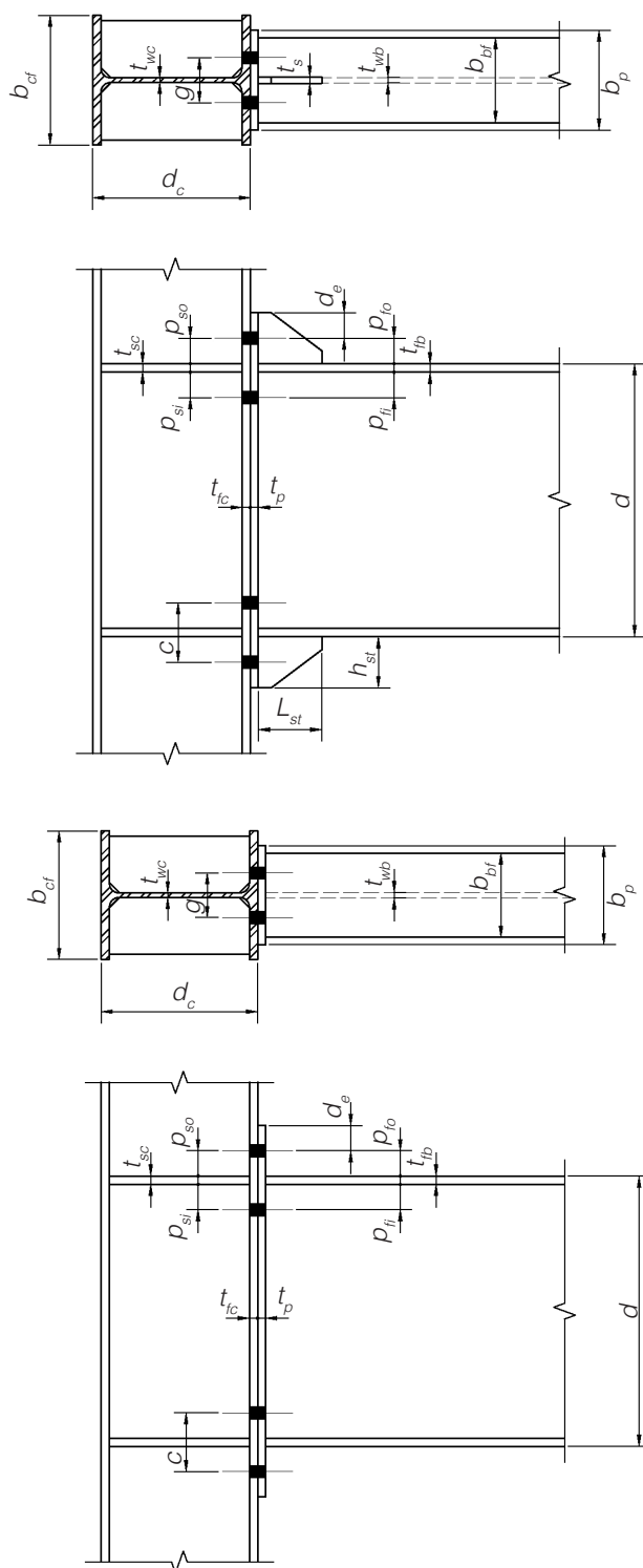
Figura B.3. Elementos principales de la conexión de placa extrema (a) rigidizada (BSEEP) y (b) sin rigidizar (BUEEP).
