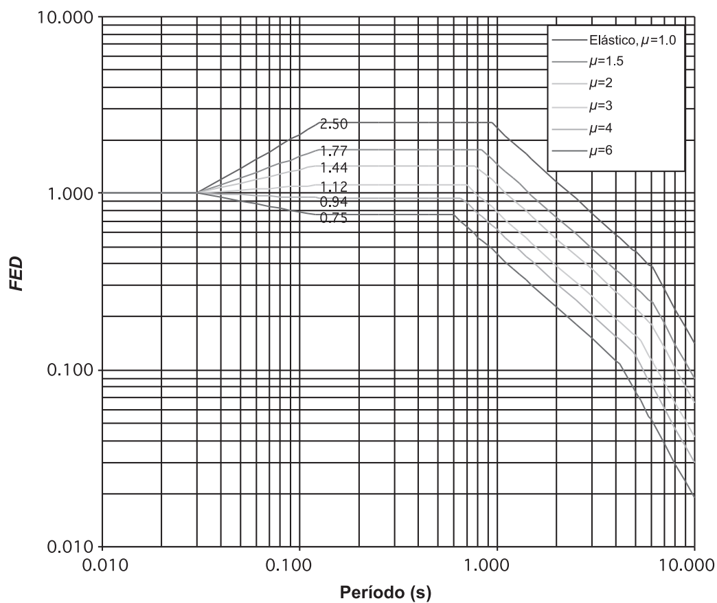
FIGURA 5.8. Factor espectral dinámico, FED , para sitios de cimentación tipo S_4 en zona sísmica III (amortiguamiento \zeta = 5\% ; ductilidades \mu = 1, 1.5, 2, 3, 4, 6 ).
